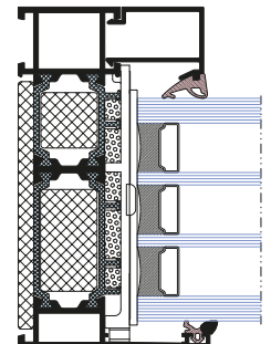
Przekrój ościeznicy okna stałego
